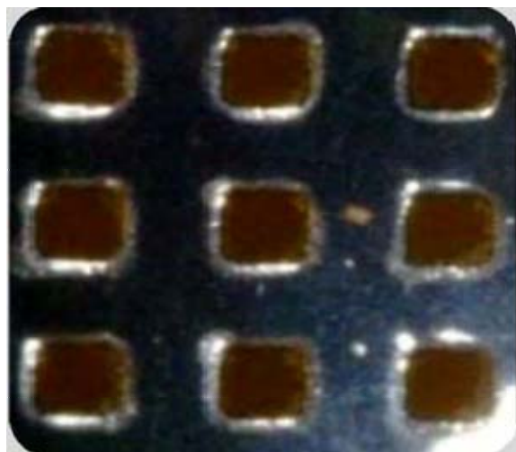
使用NanoClear®处理的模板，40次印刷后
