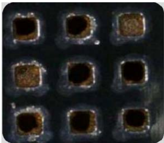
未处理的模板，14次印刷后
